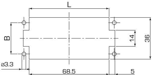
DIMA DI FORATURA PANEL CUT OUT
